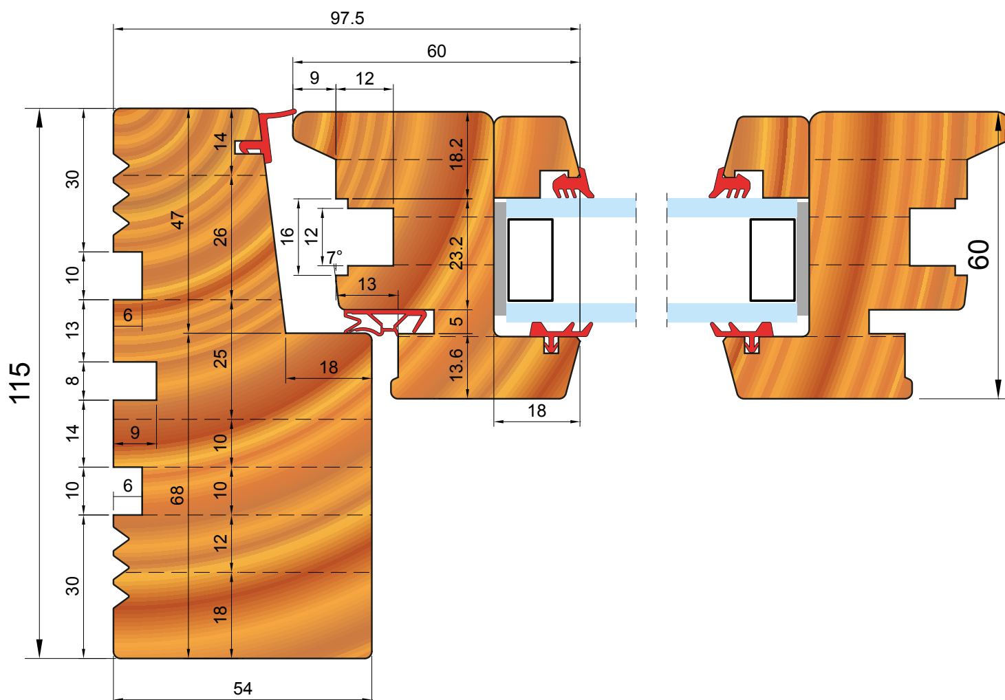
FÉLFA VÍZSZINTES METSZET HORIZONTAL SECTION JAMB
