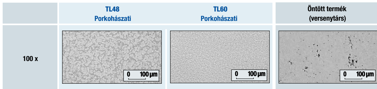
1. ábra: Porkohászati úton előállított homogén, makropórusmentes TIGRALLOY hasonló ötvözt, de öntött termékhez képest
